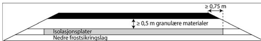
Figur 524.2 Frostsikring av veg med skumplast
