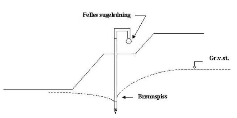
Figur 238.2 Grunnvannsenkning ved Wellpoint
