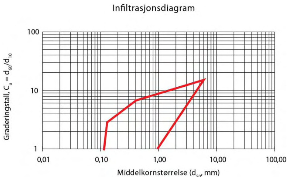
Figur 403.5 Grensekurver for anbefalte filtermasser i infiltrasjonsanlegg. Filtermasser som ligger innenfor rød grensekurve samt har d_{10} > 0,1 mm og maks 2-3 % < 0,063 mm, er tilfredsstillende.
