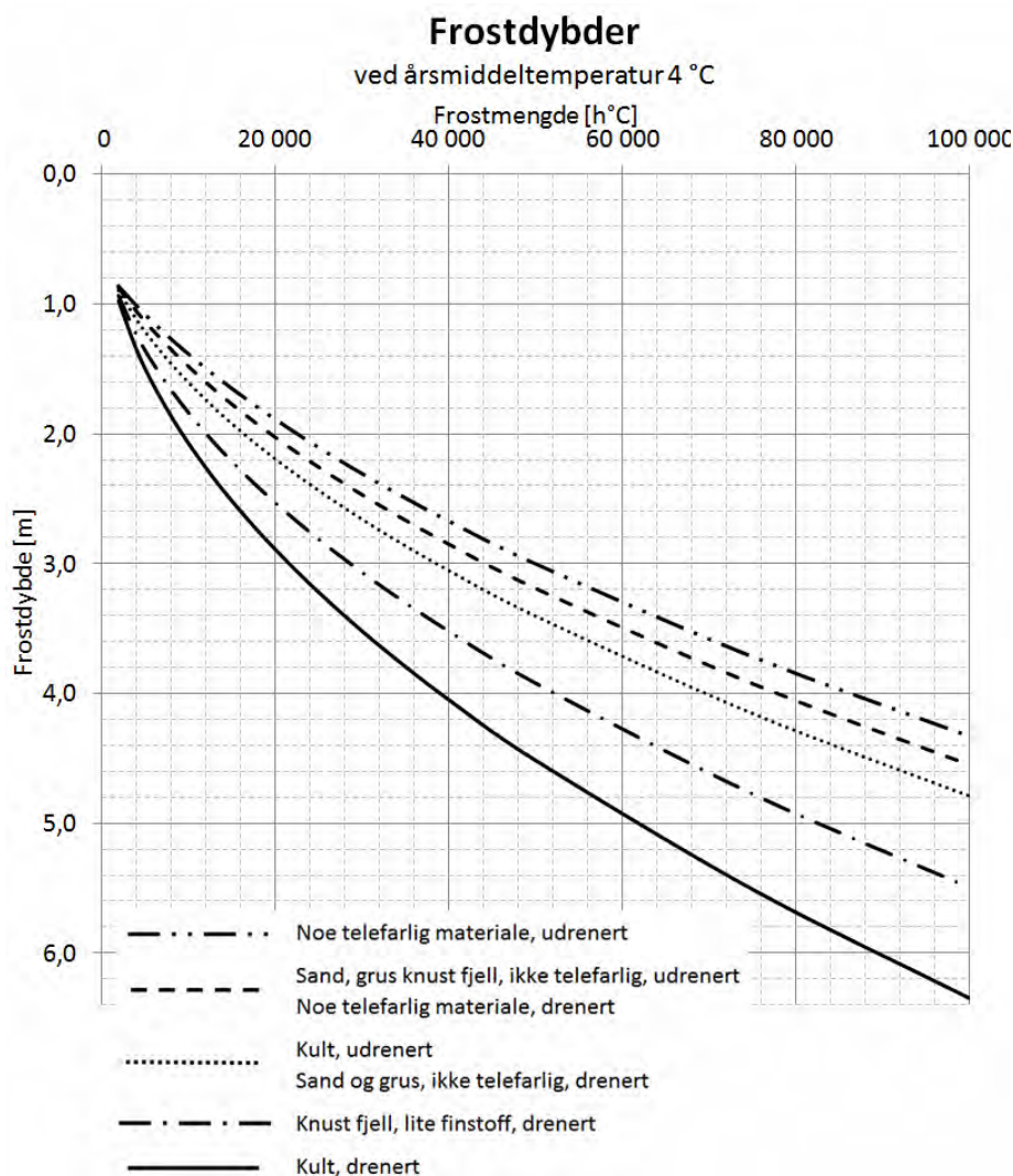
Figur 511.2 Frostdybde ved frostsikring med knust fjell, sand eller grus, årsmiddeltemperatur 4°C.
