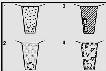
Figur 406.5 Eksempler på utforming av drenggrøft - utførelser ifølge figur 406.6.
