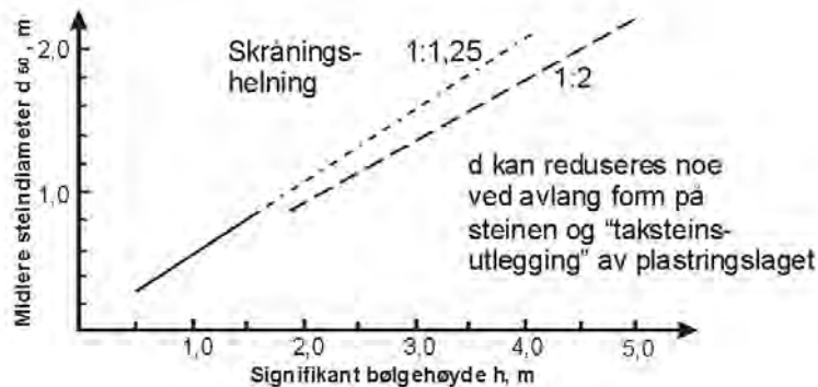
Figur 262.2 Steinstørrelse for sikring mot bølgeerosjon
