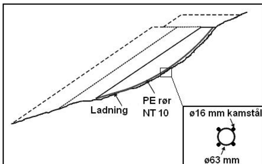
Figur 231.4 Massefortrenkning ved sprengning i plastslanger plassert på sjøbunn
