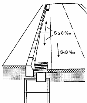
Figur 406.10 Pendelrenne
