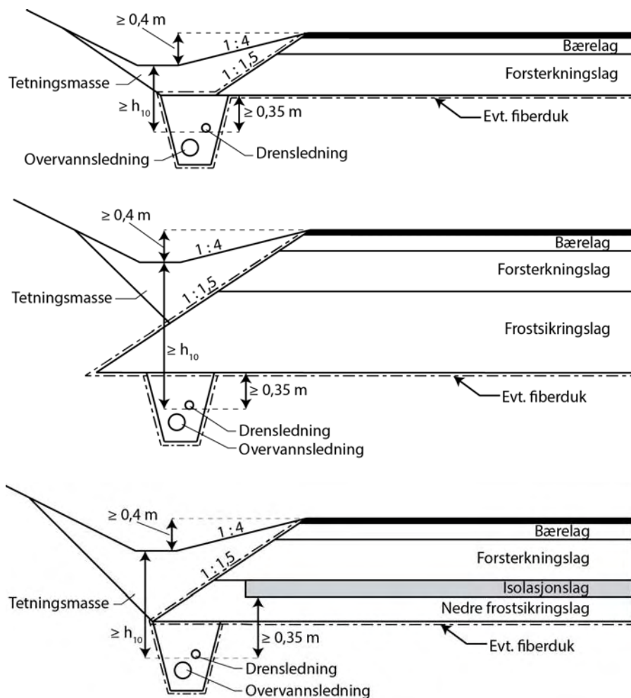
Figur 406.4 Grunne overvannsgrofter og lukket drenering
