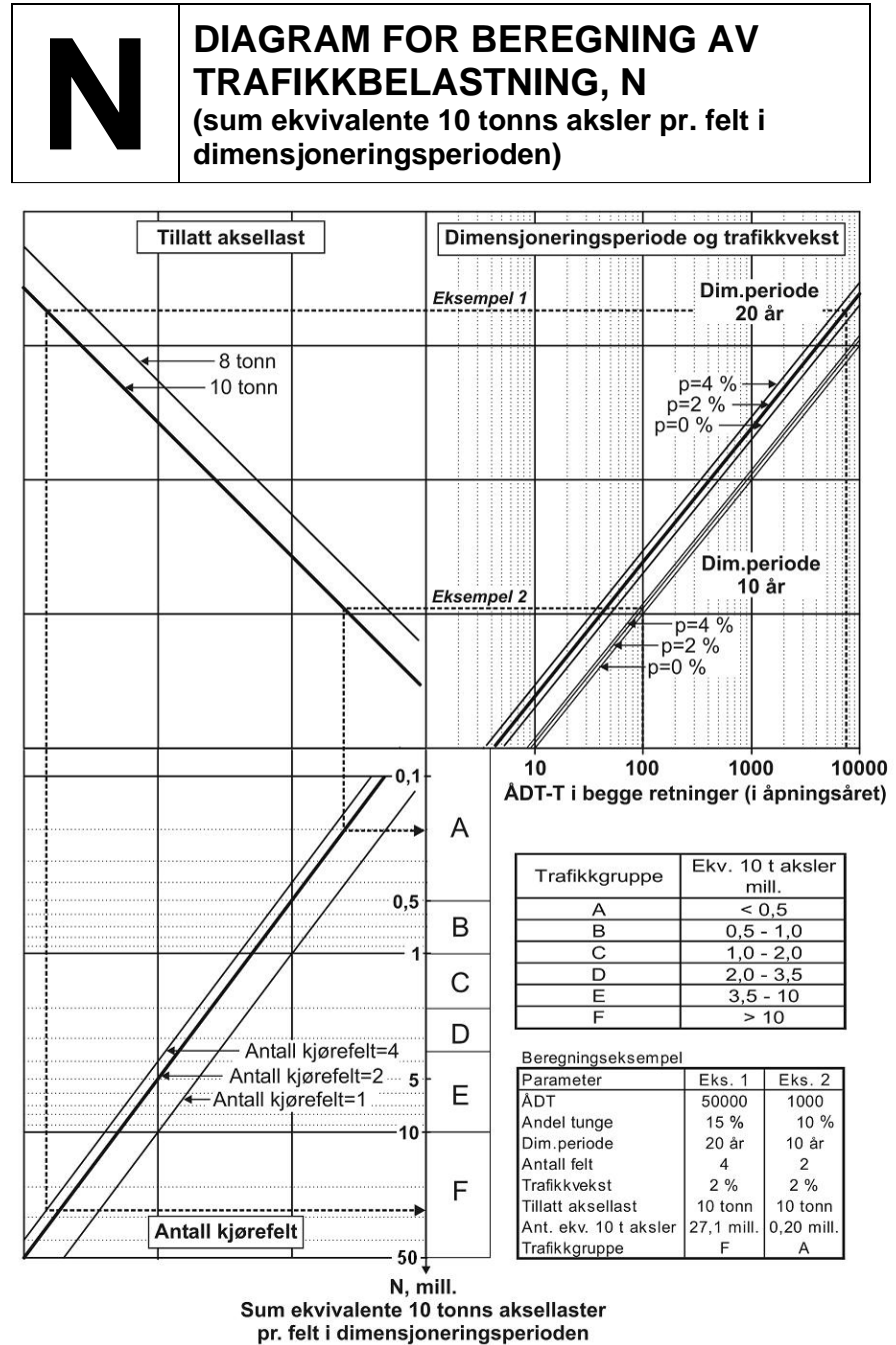
Figur 510.2 Beregning av trafikkbelastning, N
