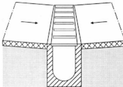
Figur 406.12 Kasserenne
