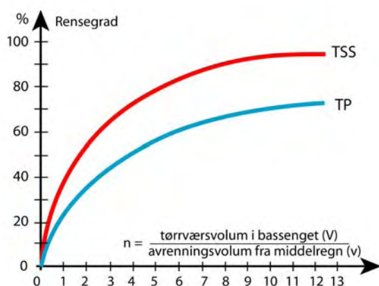
Figur 403.3. Sammenheng mellom volumfaktor ( n ) og rensegrad (%) for ulike typer forurensning, TSS (suspendert stoff, partikkelmengde) og TP (total fosformengde). 1 mm nedbør gir avrenningsvolum 10 m 3 pr. redusert ha.
