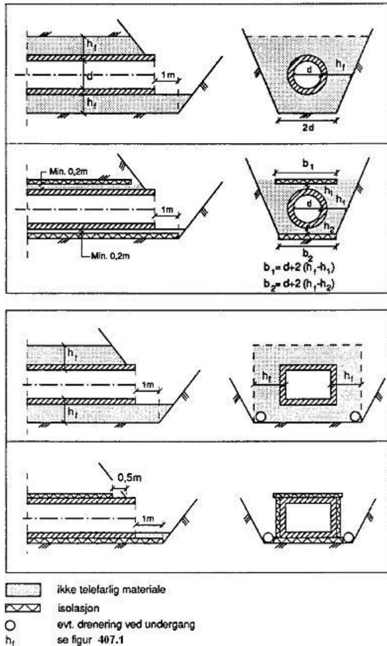
Figur 407.2 Frostsikring av underganger og kulverter/stikkrenner
