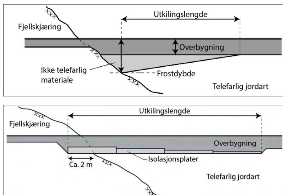
Figur 512.3 Utkiling ved overgang fjellskjæring/telefarlig grunn eller underbygning
