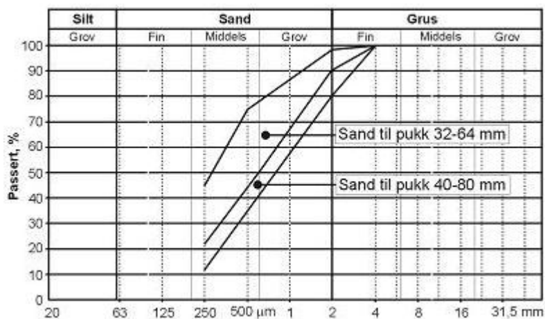
Figur 523.25 Grensekurver for sand til sementstabilisert pukk
