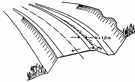
Figur 406.11 Kneking av skulder i kurve.
