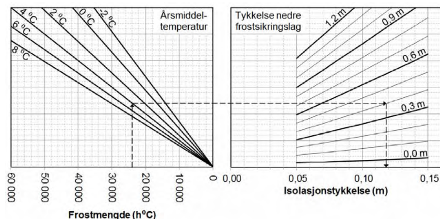
Figur 511.6 Frostmessig dimensjonering med XPS
