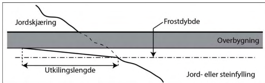
Figur 512.4 Utkiling ved overgang jordskjæring/fylling
