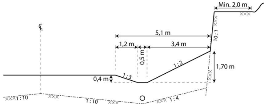
Figur 225.1 Normalprofil i bergskjæring når rekkverk ikke benyttes.
