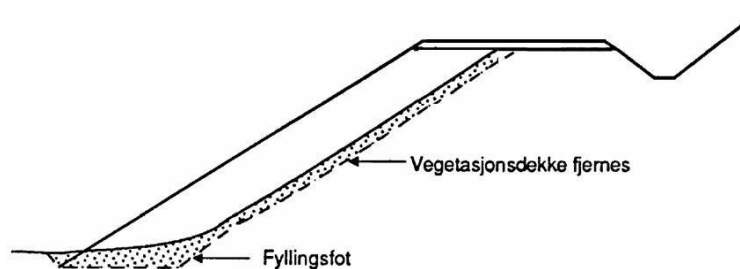
Figur 257.1 Breddeutvidelse av veg
