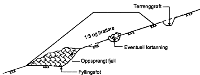
Figur 253.2 Fortanning ved berghelning 1:3 og brattere
