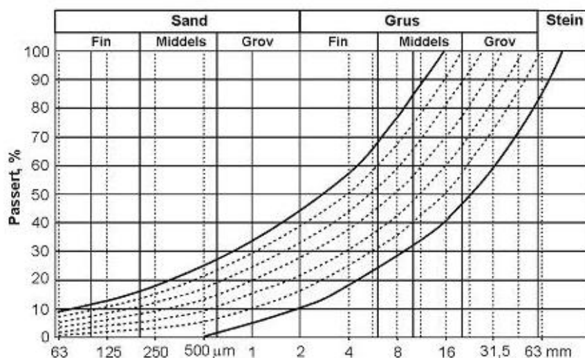
Figur 523.17 Grensekurver, Ak til bærelag og forsterkningslag
