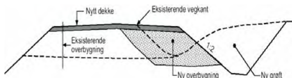
Figur V9.5 Eksempel på ensidig breddeutvidelse
