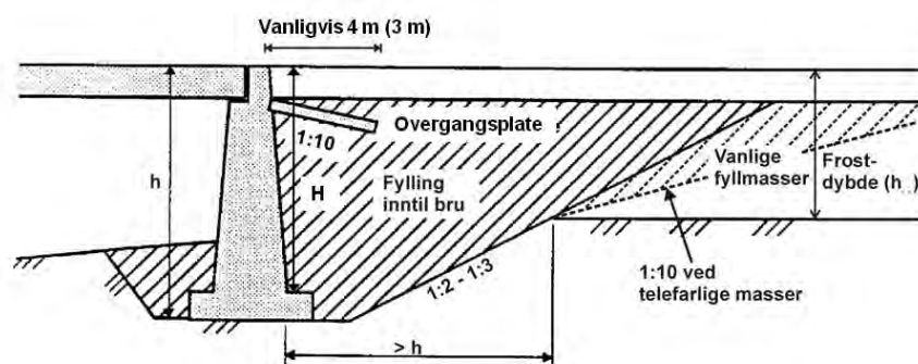
Figur 258.1 Fylling inntil bruer
