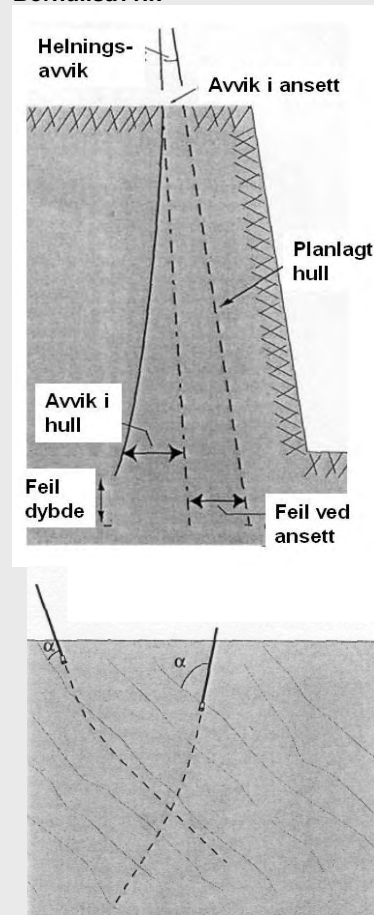
Figur 226.1 Hvis \alpha er større enn \sim 15^\circ vil borhullet bøyes mot normalen til foliasjonsretningen. Hvis \alpha er mindre enn \sim 15^\circ vil borhullet bøyes langs foliasjonsretningen.
