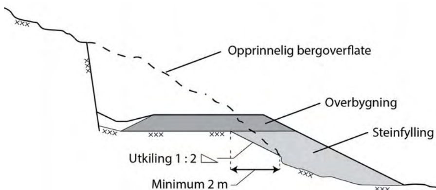
Figur 256.2 Utkiling i overgang mellom steinfylling og bergskjæring
