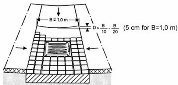
Figur 406.13 Grunn overflaterenne for åpne plasser
