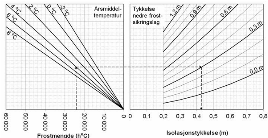
Figur 511.4 Frostmessig dimensjonering med lettklinker eller skumglass
