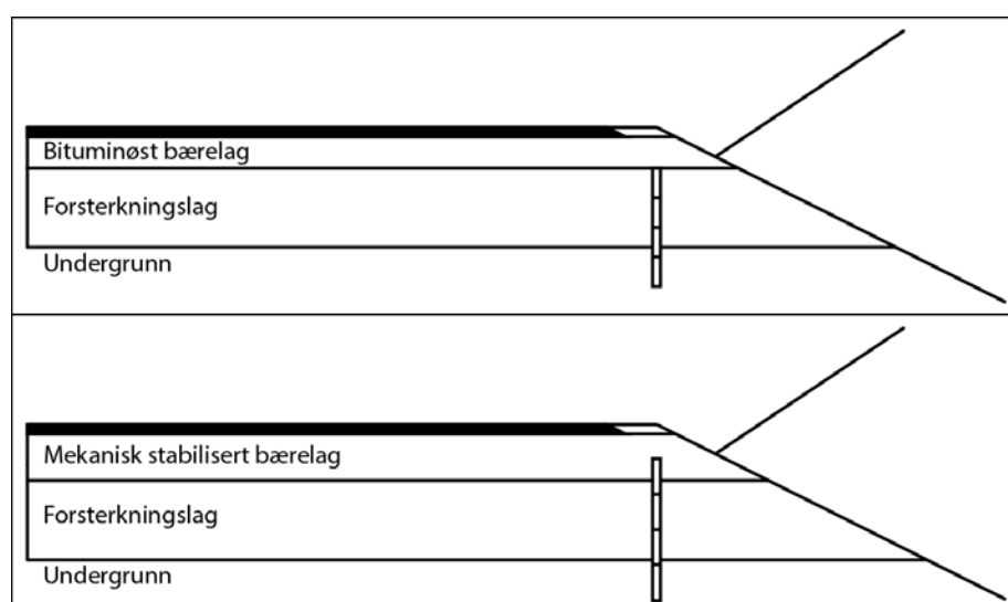
Figur 433.3 Anbefalt plassering av drensmatte ved kantdrenering
