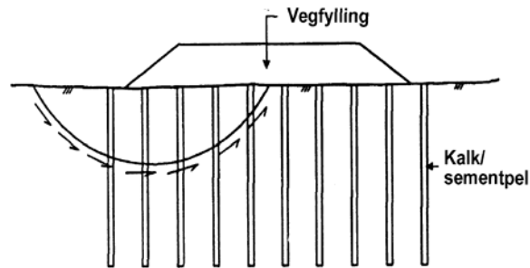
Figur 237.1 Stabilisering og/eller setningsreduksjon med kalk/semmentpeler. Ved stabilisering benyttes det gjerne geonett eller annen armering i tillegg til pelene.
