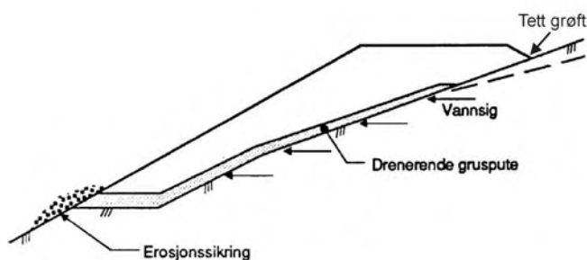
Figur 254.1 Gruspute under fylling i tverrskrånende terreng
