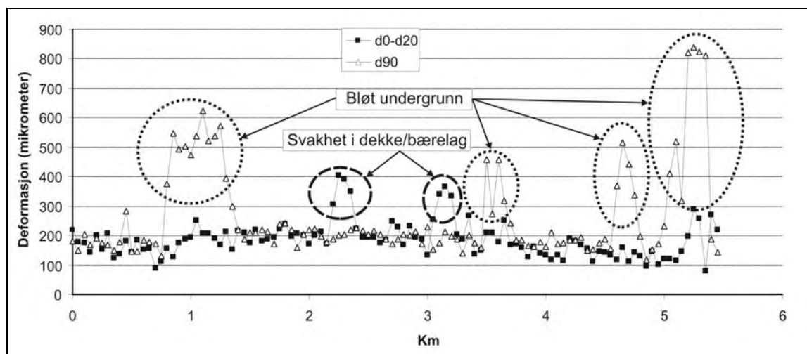
Figur V6.2 Eksempel på tolking av falloddmålinger mht. lokalisering av svake lag (d90 = nedbøyning i avstand 90 cm fra lastsentret, d0-d20 = differanse mellom nedbøyning rett under lastsentret og nedbøyning 20 cm fra lastsentret, dvs. krumning av overflaten under lastsentret)
