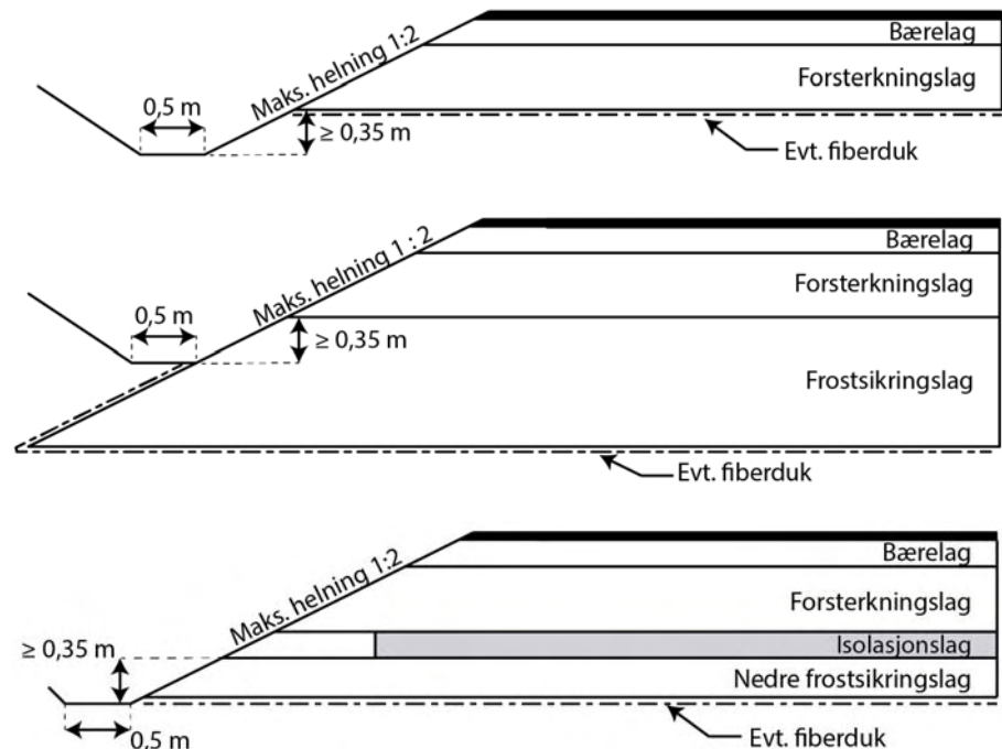
Figur 406.3 Åpen drenggrøft ved ulike overbygninger
