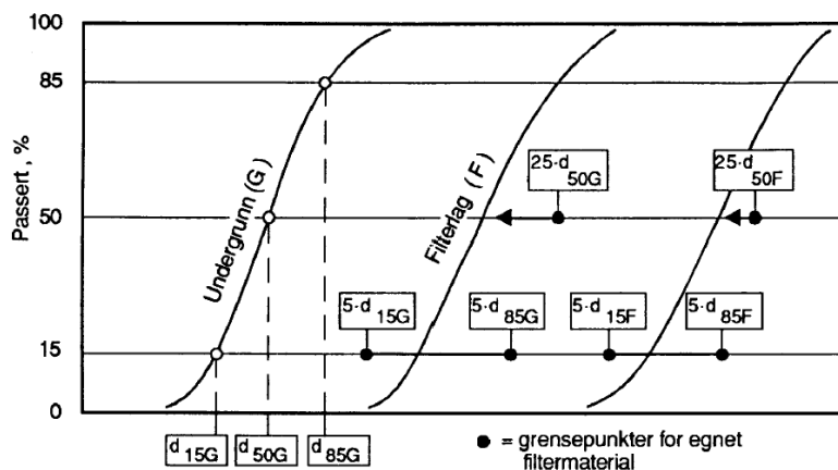
Figur 521.4 Valg av filtermateriale ut fra filterkriteriene.
