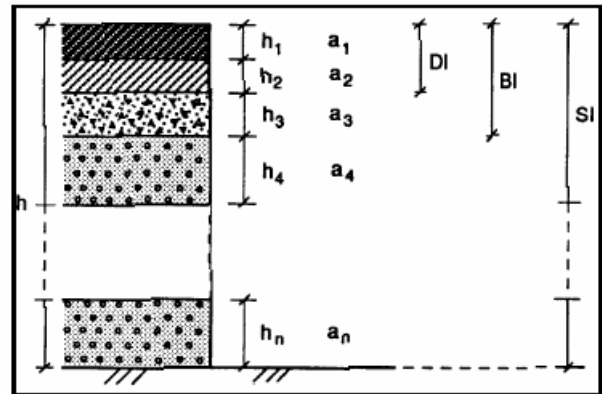
Figur V4.1 Betegnelser som nyttes i indeksmetoden
