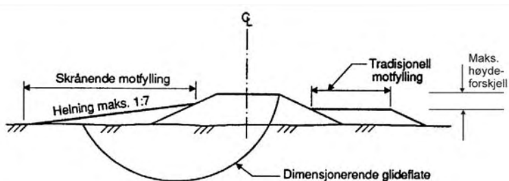
Figur 233.1 Nyttverdi av motfyllingsområde bør vurderes ved utforming
