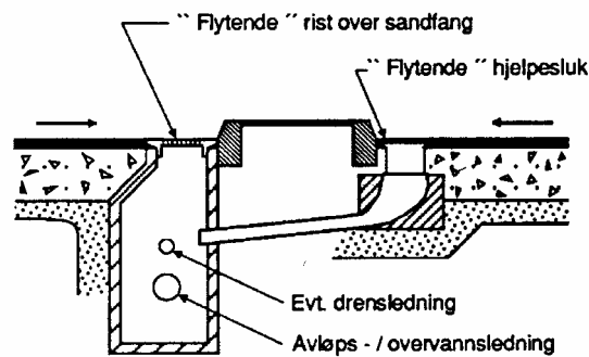
Figur 463.4 Kum med hjelpesluk
