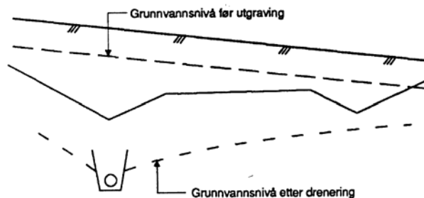
Figur 238.1 Grunnvannsenkning ved drenering
