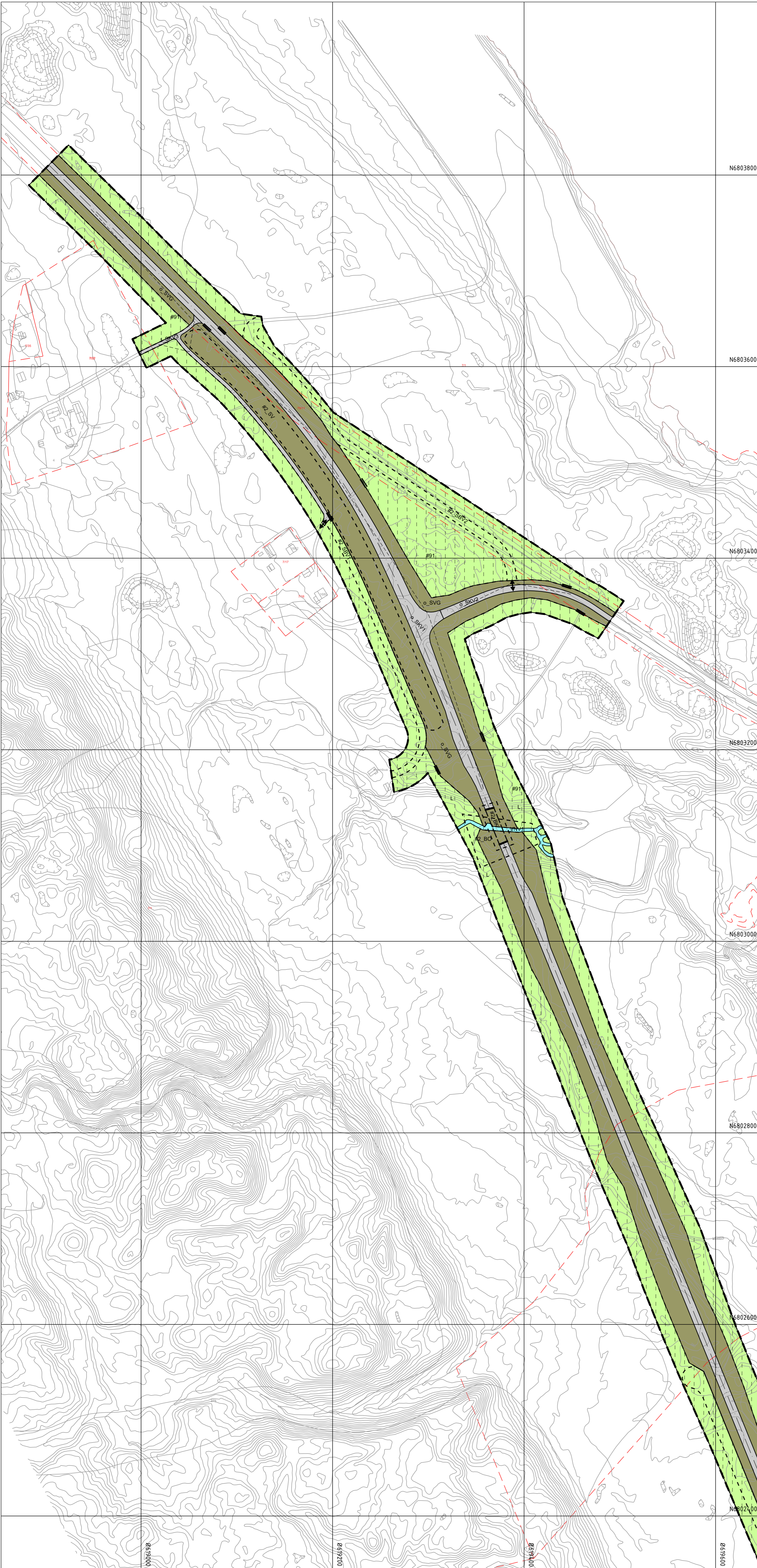
Vertikalnivå 3 - Ørtjørbekken bru (1:1000)
