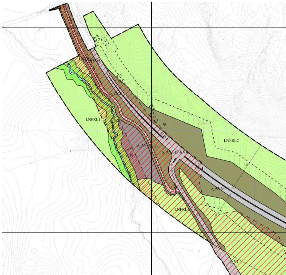
Figur 14 Utsnitt av reguleringsplanen for midlertidig løsning av koblingen mellom prosjektene Retvet - Vinterbro og Knapstad – Retvet.
