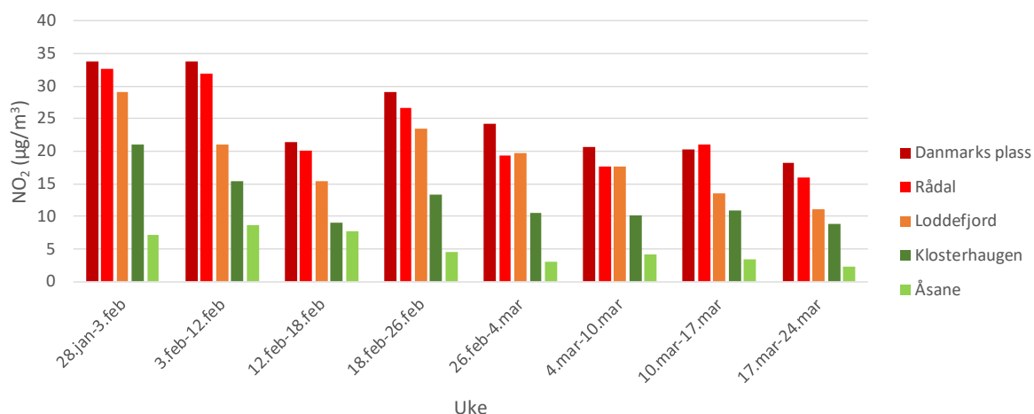
Figur 17: \text{NO}_2 -konsentrasjon ved målestasjoner i Bergen, midlet over de enkelte eksponeringsperiodene for passive prøvetakere plassert ved E16 Gaupås. Danmarks plass, Rådalen og Loddefjord er veinære stasjoner; Klosterhaugen og Åsane er bakgrunnsstasjoner.
