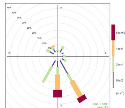
Figur 7: Fordeling av vindretning og vindhastighet (vindroser) på E39 Vågsbotn (venstre) og på Gaupås (høyre) for de enkelte eksponeringsperiodene. Figurene viser med hvilken frekvens det forekommer vind fra angitt retning. Vindmåling på Gaupås startet 6. februar.
