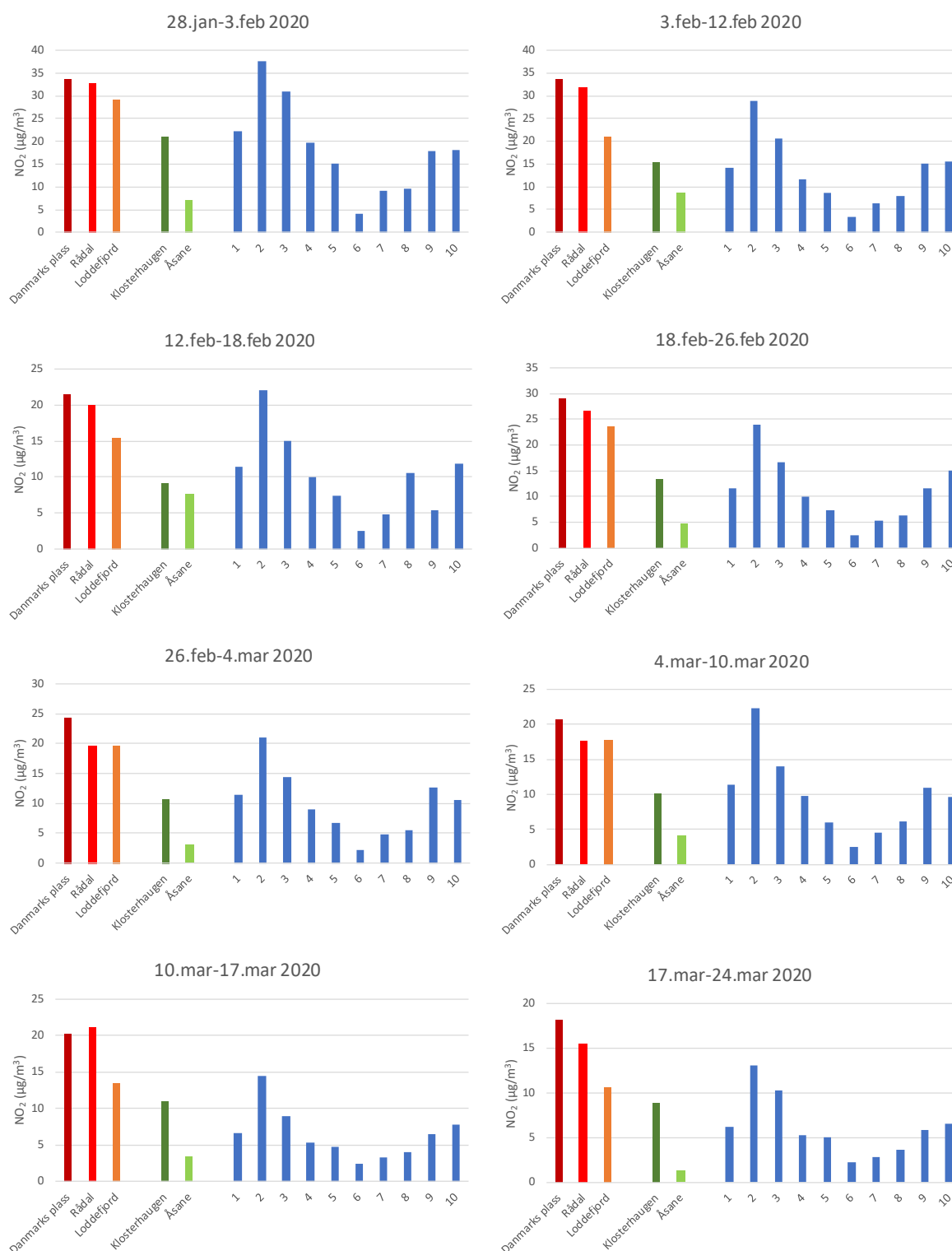
Figur 18: Sammenligning av NO 2 -konsentrasjonen i måleområdet (prøvetakere 1 – 10) med NO 2 -nivået ved målestasjoner i Bergen for hver eksponeringsperiode.
